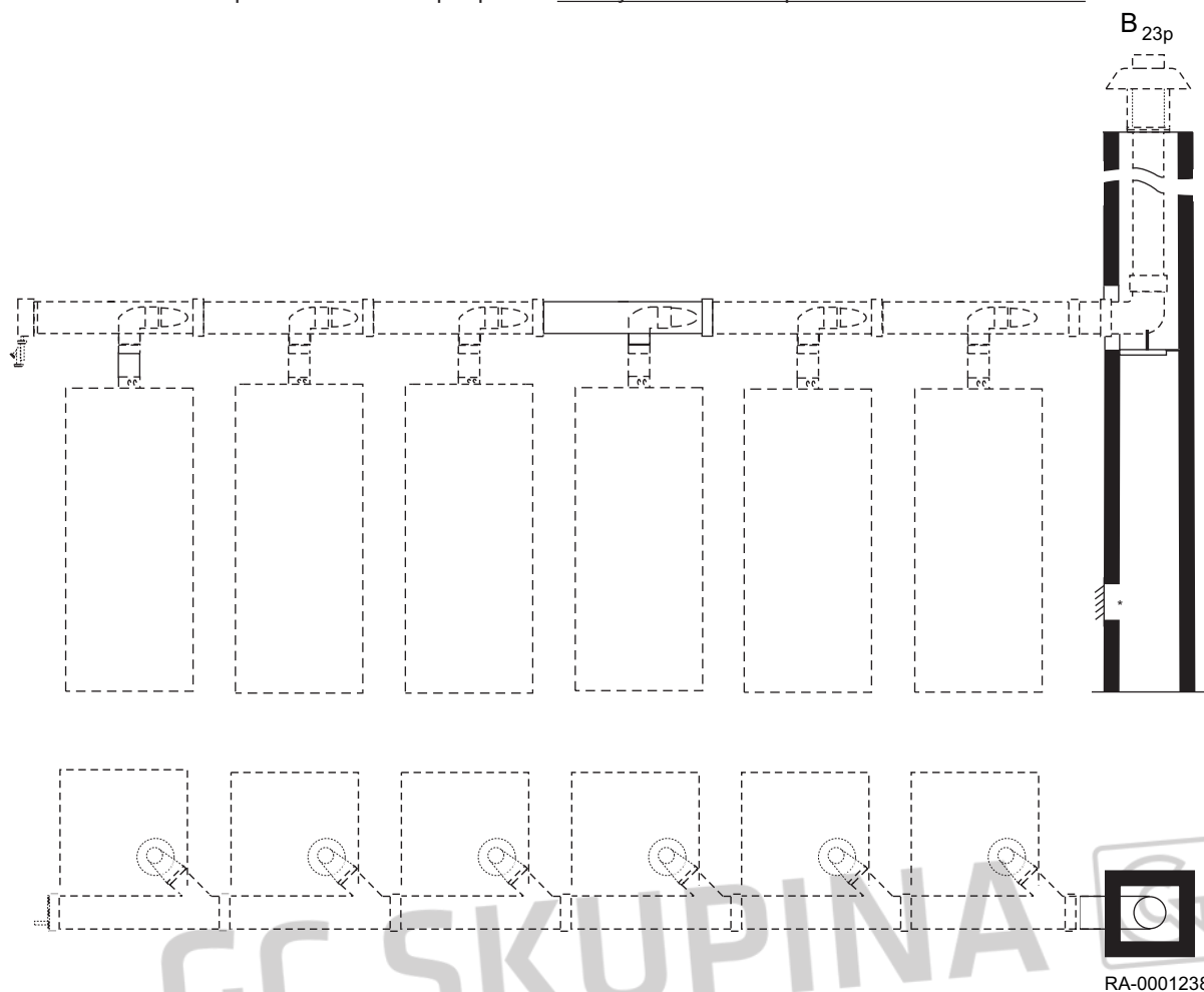
Obr.17 Soustava spalínového vedení pro provoz závislý na vzduchu z prostoru instalovaného kotle
