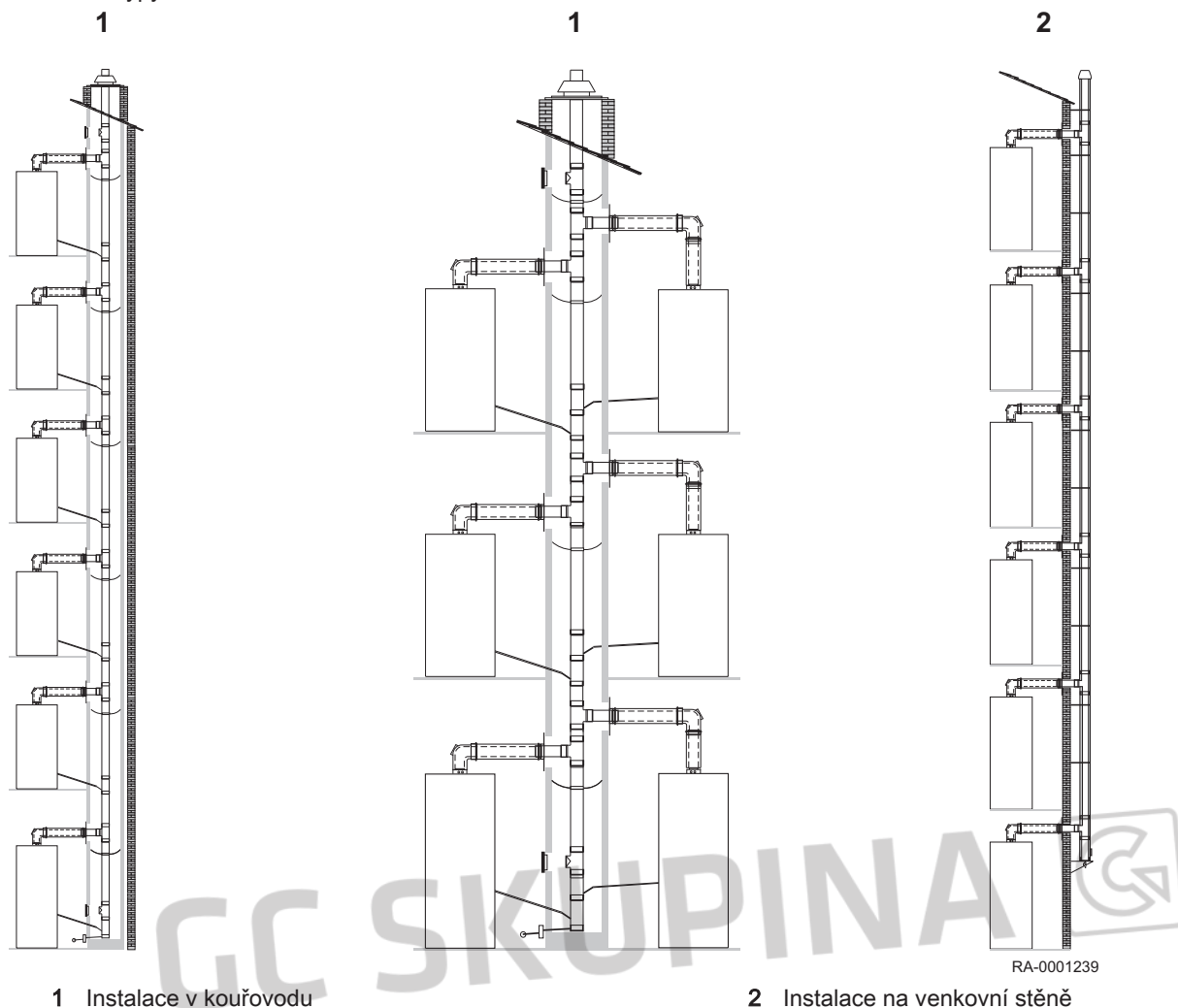
Obr.19 Typy soustav
