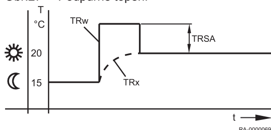
Obr.27 Podpurné topení
