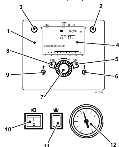
Obr.5 Provozní prvky
